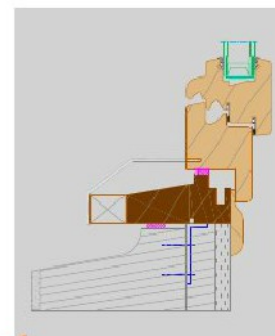
Coupe verticale
